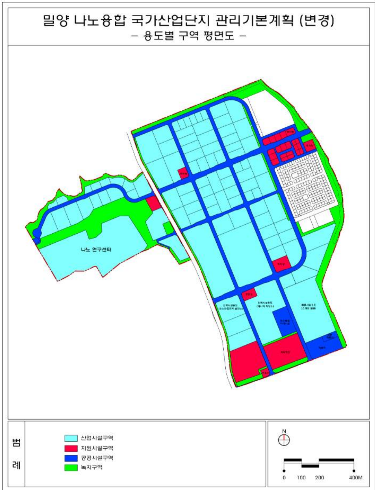
(별첨 #1) 밀양 나노융합 국가산업단지 용도별 구역 평면도
